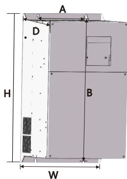
图7-2 JL950系列 钣金结构外型尺寸及安装尺寸示意图
