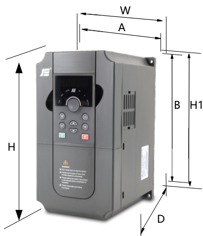
图7-1 JL950系列 塑胶结构外型尺寸及安装尺寸示意图
