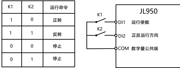
图6-7 两线式模式2
