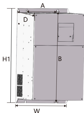
图7-2 JL930系列 钣金结构外型尺寸及安装尺寸示意图
